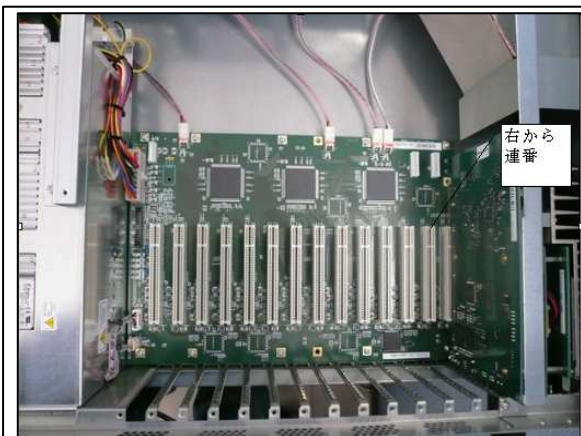
拡張スロット部 マザーボード写真
