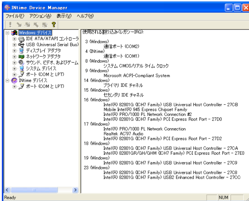
INtime Device Configuration上 デバイス表示
