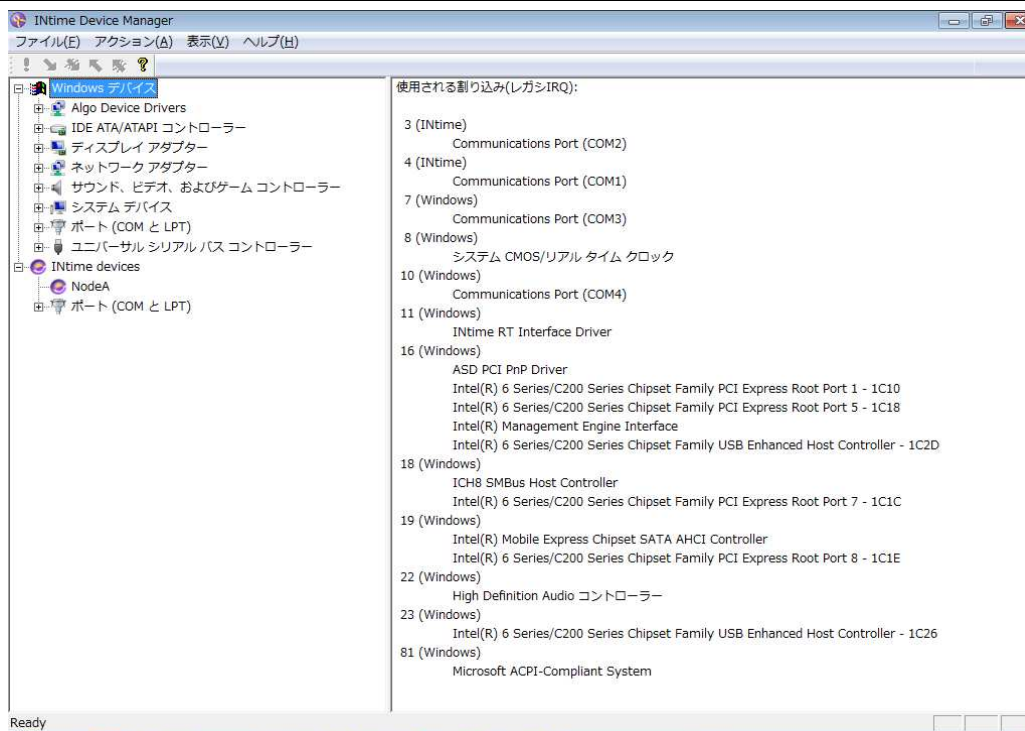
INtime Device Configuration上 デバイス表示
