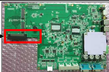
拡張スロット部 マザーボード写真
